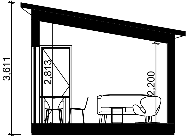
SEKTION
