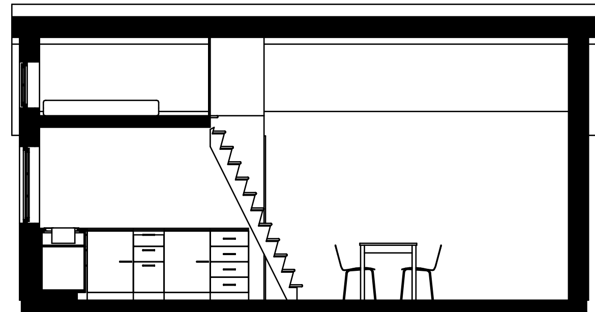
SEKTION
