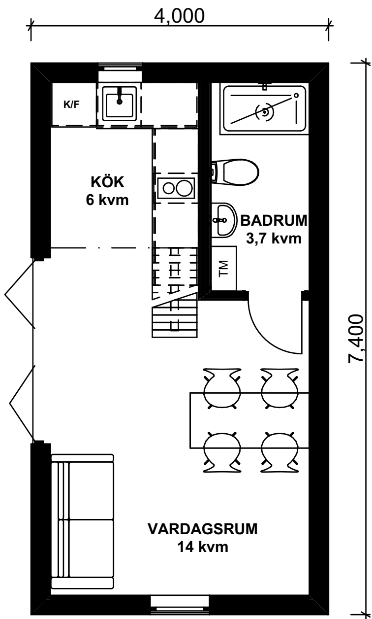
PLAN BYA: 29,9 kvm
