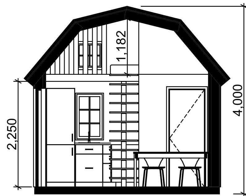
SEKTION
